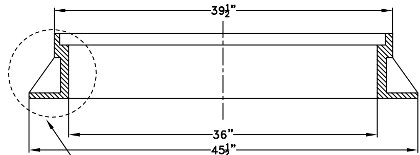
MANHOLE FRAME
